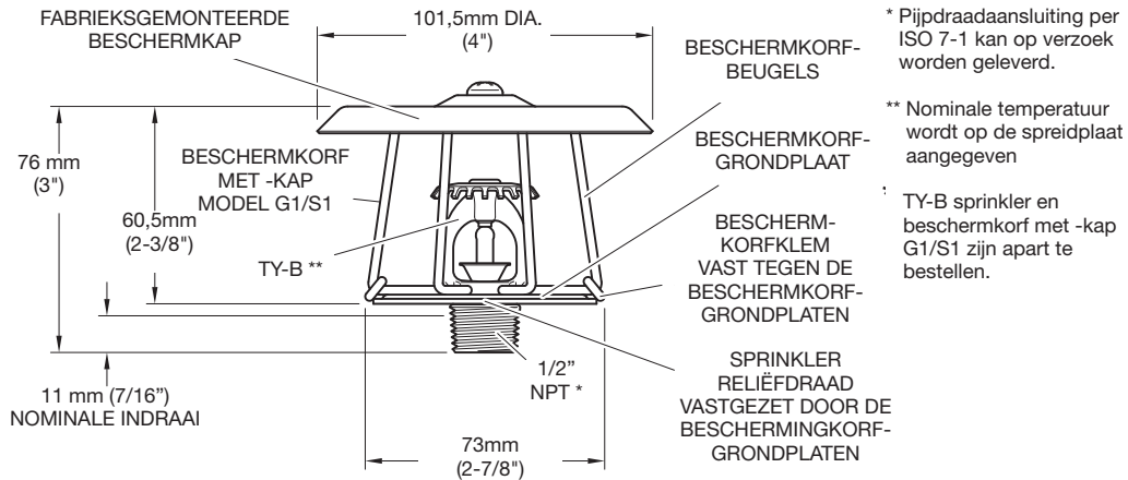
FIGUUR 1 SERIE TY-B STAANDE (TY315 STELLING SPRINKLERS MET G1/S2 BESCHERMKORF EN -KAP
