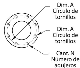
— ESPECIFICACIÓN Y DIMENSIONES PARA LA PERFORACIÓN DE BRIDAS
