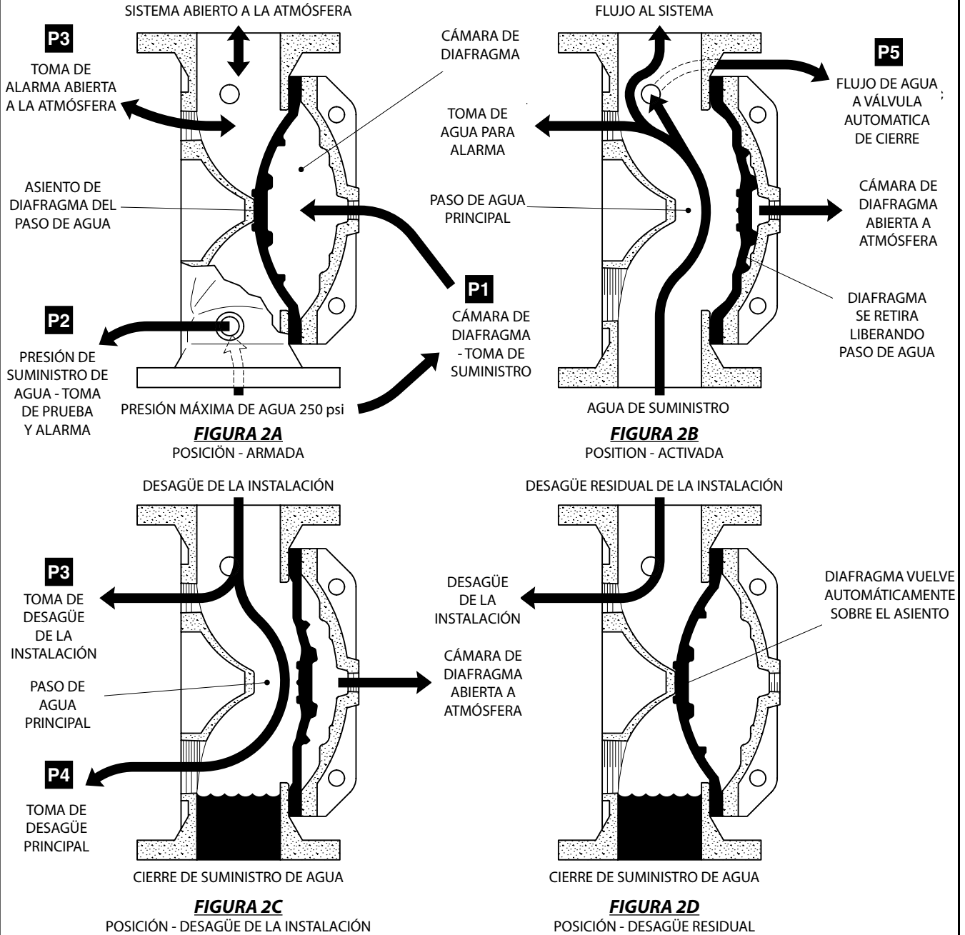
FIGURA 2 VÁLVULA DE DILUVIO MODELO DV-5, 1-1/2" a 8" (DN40 a DN200) — VÁLVULA ARMADA Y ABIERTA —
